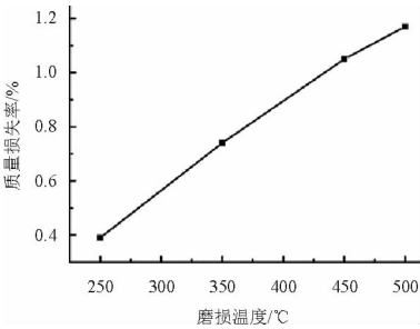
图 8 不同温度条件下堆焊层的质量损失率 Fig.8 The weight loss rate of Stellite6 overlay at different temperatures
