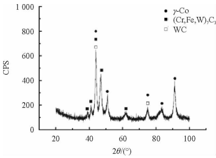
图 2 Stellite6 堆焊层 XRD
