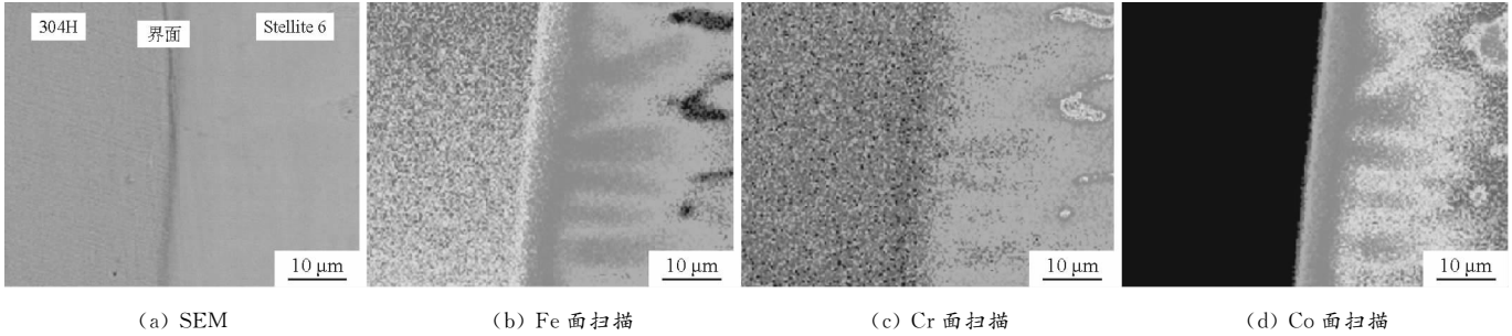
图 4 Stellite6 堆焊层 SEM 形貌及元素面扫描
