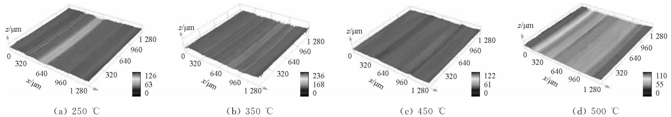
图 10 不同温度堆焊层磨损面形貌
