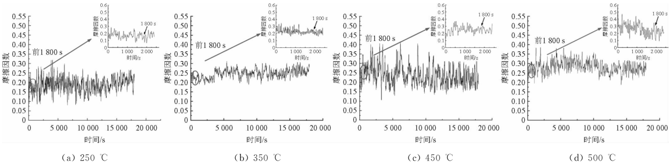
图 7 不同温度对堆焊层摩擦因数的影响
