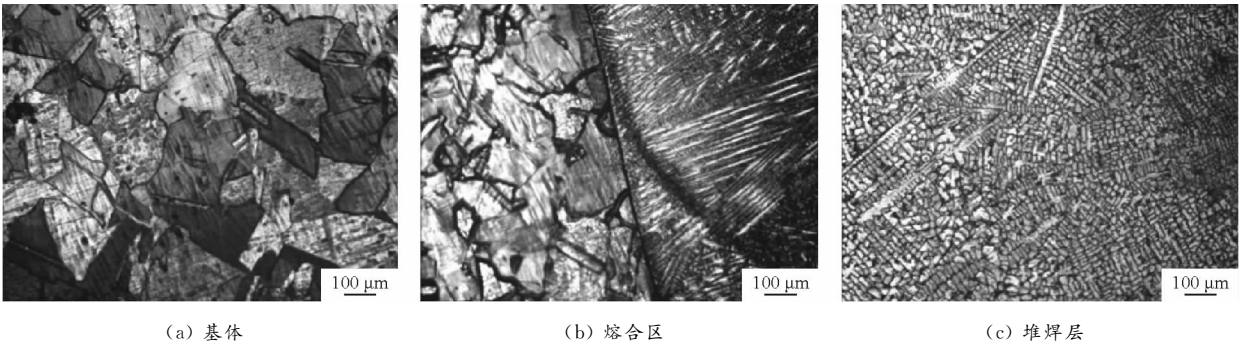
图 1 Stellite6 钴基合金堆焊层微观组织
