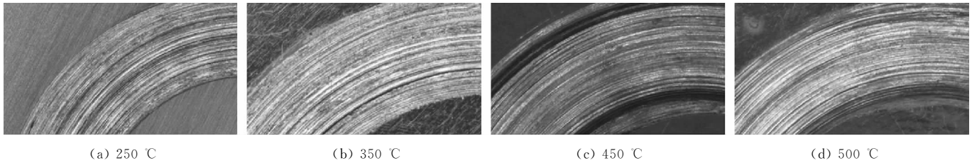
图 9 不同温度下堆焊层磨损面形貌
