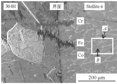
图 3 Stellite6 堆焊层元素分布
