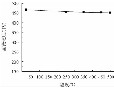
图 6 不同温度保温 5 h 堆焊层硬度变化
