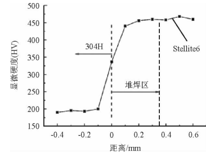
图 5 基体到 Stellite6 堆焊层硬度变化情况
